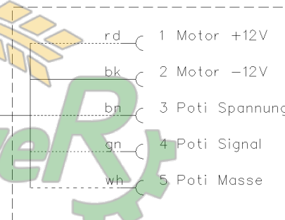
Aktuator rechts
