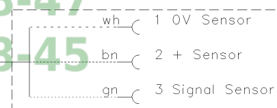
Füllstandsensor rechts
